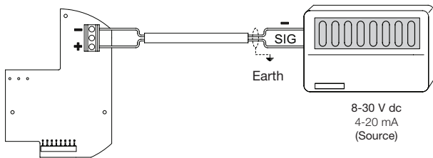
Xgard Type 2 PCB
